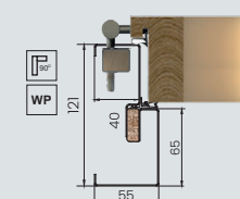
stalowa NT/75
