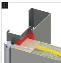
1 Wypełnienie skrzydła panel akustyczny
