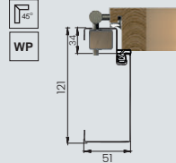
alumiowy ALU 15/54
