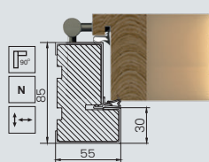
drewniano-stalowa DS/75, DS/75 N
