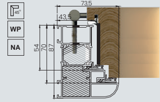
aluminiowa ALU/90
