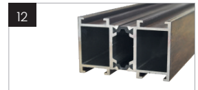
Poszerzenie aluminiowe boczne/ górne do ościeznicy: ALU/54 • 35 mm (1) • 50 mm (2)
