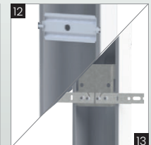
Elementy wzmocniające konstrukcję ościeżnicy z kotwami montażowymi lub bez 12. Ościeżnica 10/54, 11/54 13. Ościeżnica 15/54
