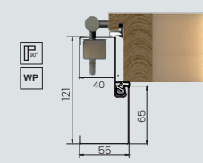
stalowa S15/75
