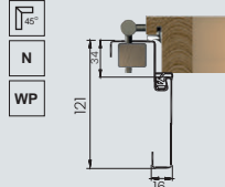
alumiowy ALU 11/54, ALU 11/54 N
