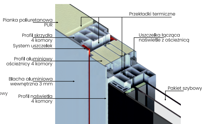
PROFIL OŚCIEŻNICY
