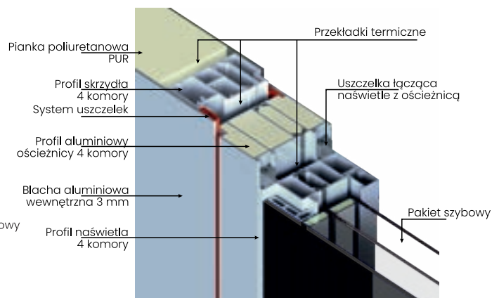
PROFIL OŚCIEŻNICY
