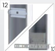
12 Elementy wzmacniające konstrukcję ościeżnicy z kotwami montażowymi lub bez 13 Ościeżnica 10/54,11/54 13. Ościeżnica 15/54
