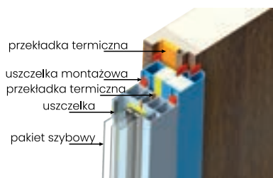
PROFIL NAŚWIETLA PROFIL OŚCIEŻNICZY ALU/90
