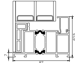
PROFIL NAŚWIETLA
