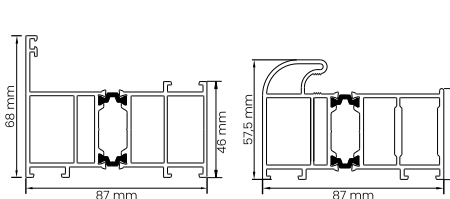
PROFIL NAŚWIETLA PROFIL OŚCIEŻNICZY ALU/75
