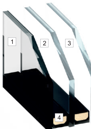
BUDOWA PAKIETU SZYBOWEGO:
