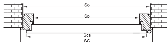
Drzwi trzy przylgowe 3P
