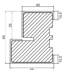
Ościeżnica drewniano-stalowa DS/54
