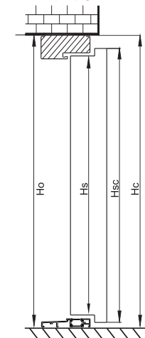
Drzwi cztery przylgowe 4P
