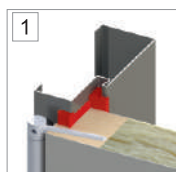
Wypełnienie skrzydła PŁYTA SKALNEJ WEŁNY MINERALNEJ
