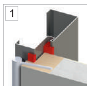
Wypełnienie skrzydła SPIENIONY POLISTYREN
