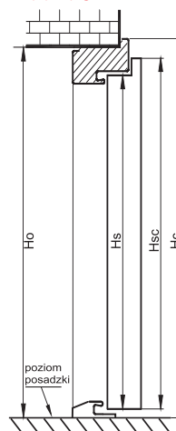
Drzwi trzy przylgowe 3P
