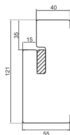
Ościeżnica stalowa NT/54, NT/54 AKU
