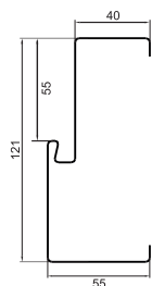
Ościeżnica stalowa S15/75
