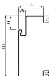
Ościeżnica stalowa S15/54
