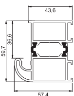
Ościeżnica aluminiowa ALU/54
