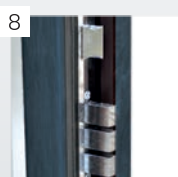
Zamek listwowy klasy 4 z blokadą klamki z zabezpieczeniem górnym i dolnym
