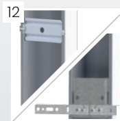
Elementy wzmacniające konstrukcję ościeznicy z kotwami montażowymi lub bez 12. Ościeznica 10/54,11/54 13. Ościeznica 15/54
