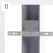
Elementy wzmacniające konstrukcję ościeznicy z kotwami montażowymi
