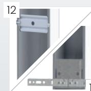
Elementy wzmocniające konstrukcję ościeznicy z kotwami montażowymi lub bez 12. Ościeznica 10/54, 11/54 13. Ościeznica 15/54
