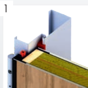
Wypełnienie skrzydła panel akustyczny
