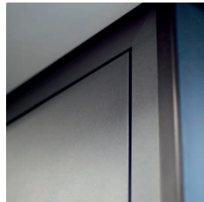
Zlicowane skrzydło z ościeżnicą
