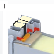
1 Wypełnienie skrzydła PIANA POLIURETANOWA
