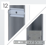
Elementy wzmacniające konstrukcję ościeżnicy z kotwami montażowymi lub bez 12. Ościeżnica 10/54, 11/54 13. Ościeżnica 15/54
