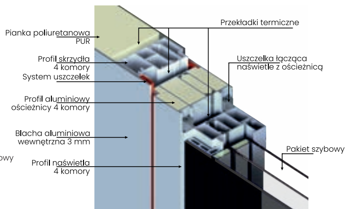
PROFIL OŚCIEŻNICY
