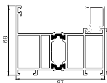
PROFIL NAŚWIETLA
