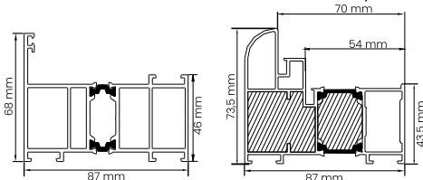
PROFIL NAŚWIETLA PROFIL OŚCIEŻNICZY ALU/90
