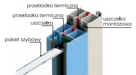
PROFIL NAŚWIETLA PROFIL OŚCIEŻNICZY ALU/54
