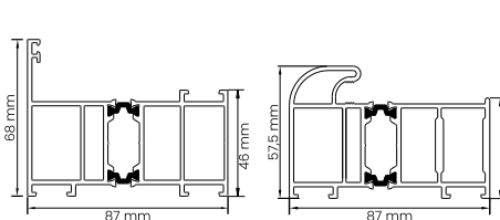
PROFIL NAŚWIETLA PROFIL OŚCIEŻNICZY ALU/75
