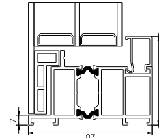
PROFIL NAŚWIETLA
