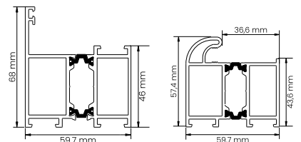
PROFIL NAŚWIETLA PROFIL OŚCIEŻNICZY ALU/54
