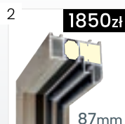
2 Ościeżnica aluminiowa ALU/90 trzykomorowa z podwójnym uszczelnieniem z przegrodą PCW wypełnioną pianą
