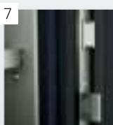
7 Zasuwnica GU Secure Automatic z blokadą klamki
